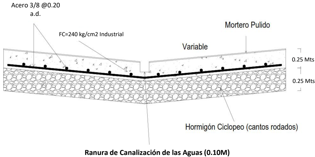
SECCION TRANSVERSAL
